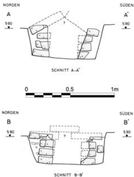
Abb. 177 F/I-o/19-Grab 4, Schnitte A-A' und B-B'
