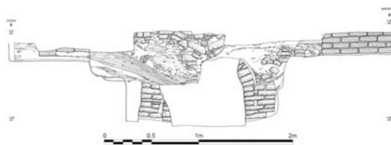
Abb. 223 F/I-p/19-Grab 1, Schnitt B-B'
