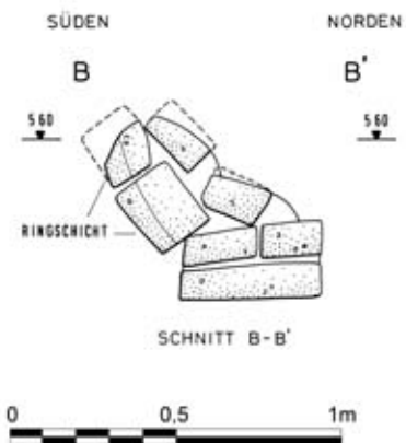
Abb. 215 F/I-p/18-Grab 4, Schnitt B-B'
