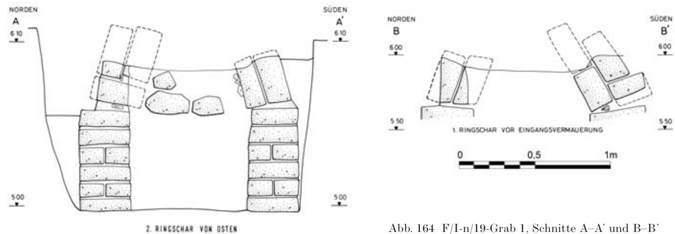
Abb. 164 F/I-n/19-Grab 1, Schnitte A–A' und B–B'
