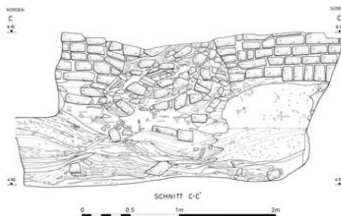
Abb. 224 F/I-p/19-Grab 1, Schnitt C-C'
