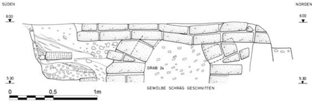
Abb. 143 F/I-m/19, Schnitt durch Gräber 10, 23, 24, 25
