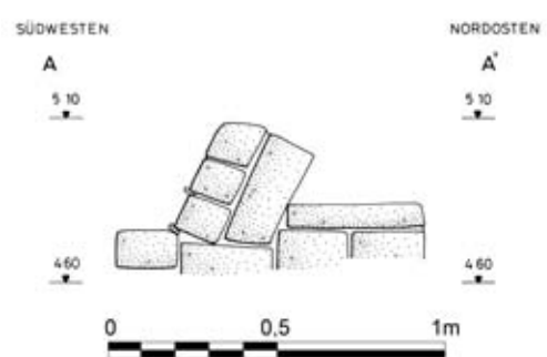
Abb. 137 F/I-1/20-Grav 54, Schnitt A–A'
