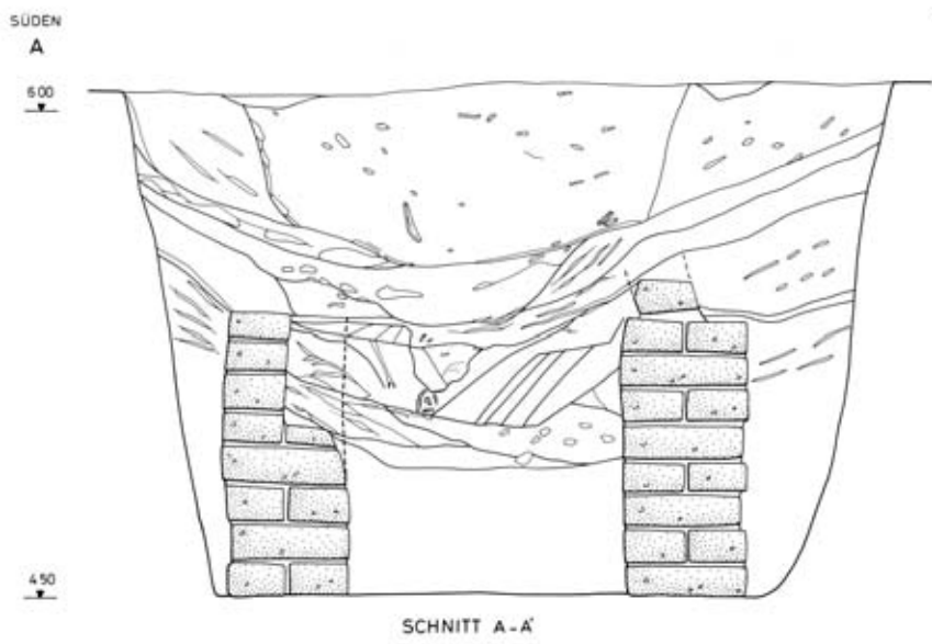
Abb. 214 F/I-p/18-Grab 4, Schnitt A-A'
