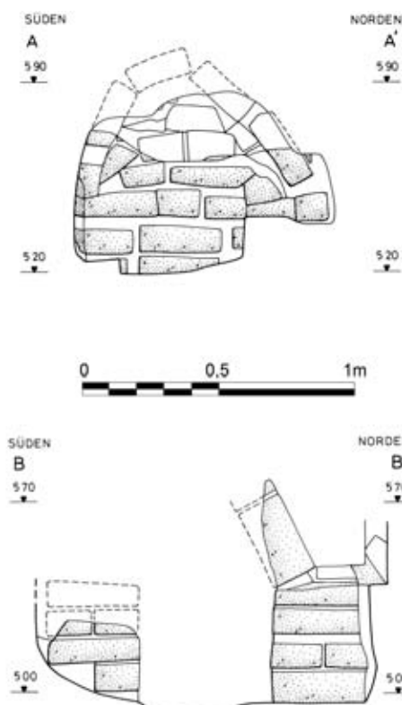
Abb. 207 F/I-o/20-Grab 14; Schnitte A–A' und B–B'
