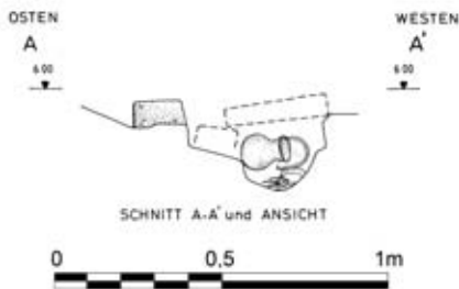
Abb. 183 F/I-o/19-Grab 6, Schnitt A–A' und Ansicht
