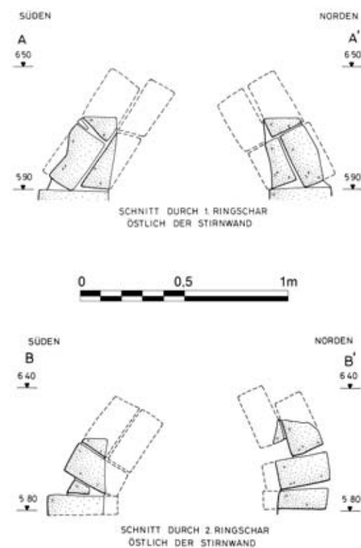
Abb. 160 F/I-n/18-Grab 7, Schnitte A–A' und B–B'
