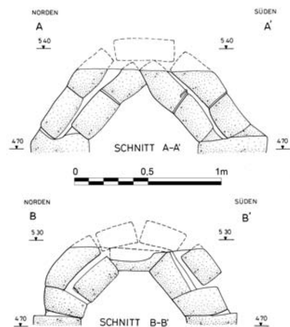
Abb. 125 F/I-j/21-Grab 13, Schnitte A–A' und B–B'
